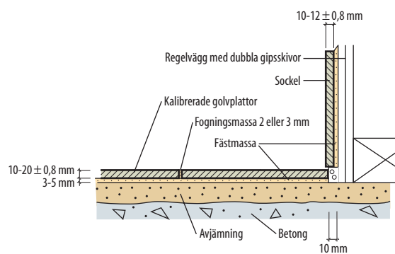
Fig 4.20 Läggningskonstruktion G3.
